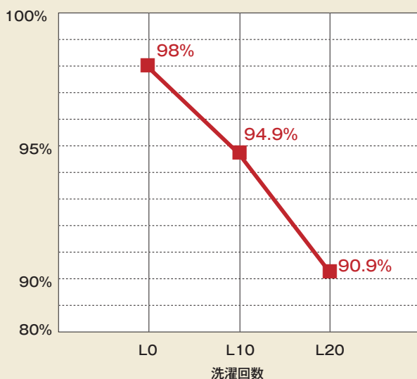
アンモニア
