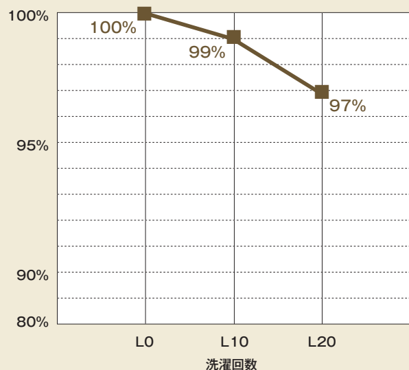
硫化水素
